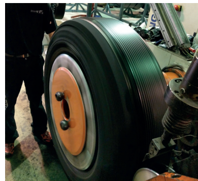
Ekstrudering av ny gummi på varmvulk.
